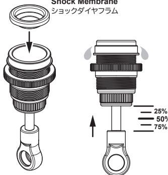
T070 Shock Membrane ショックダイヤフラム
