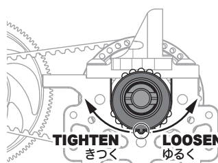
UPPER DIFF POSITION デフ位置 高
