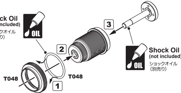
T045 Shock Shaft ショックシャフト
